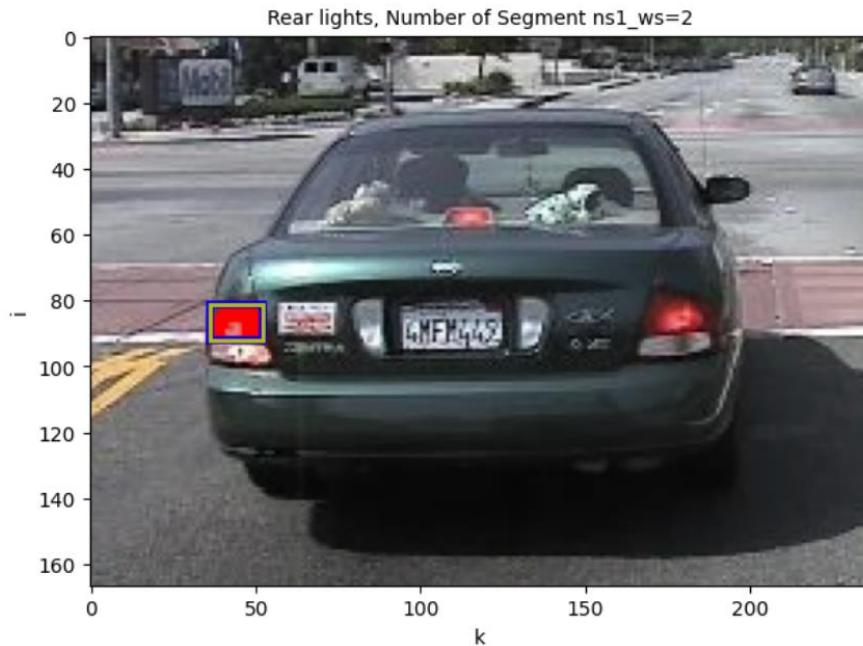
Рис. 1. Зображення з виявленим сегментом лівого ліхтаря (сегмент виділено прямокутником)
