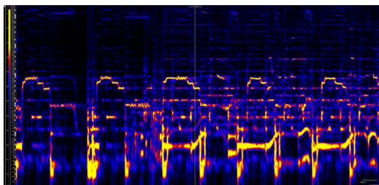
Рис. 2.2.2. Спектрограма звукового сигналу артилерійського пострілу
