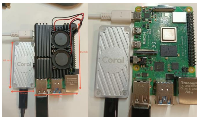
Рис. 1. (Лівий рисунок) Збірка Raspberry Pi 4 та TPU Coral USB Accelerator в захисному кейсі з двома охолоджувальними кулерами. (Правий рисунок) Збірка Raspberry Pi 4 та TPU Coral USB Accelerator без захисного кейсу
