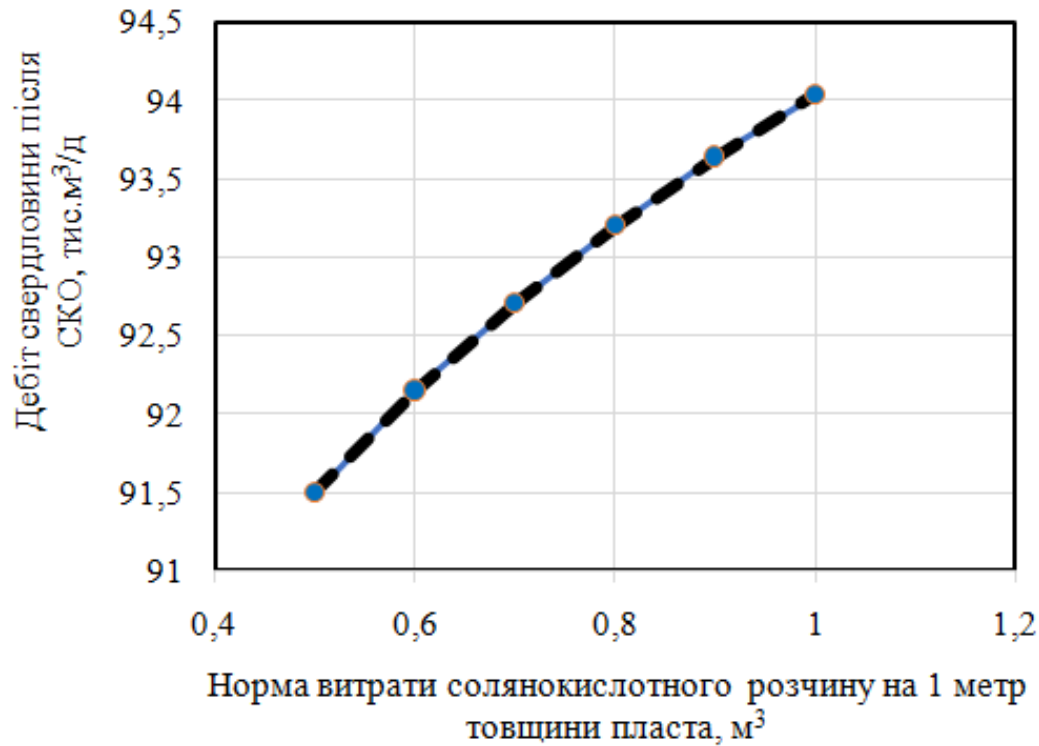
Рис 2. Залежність дебіту свердловини після проведення солянокислотної обробки від норми витрати солянокислотного розчину на один метр товщини пласта
