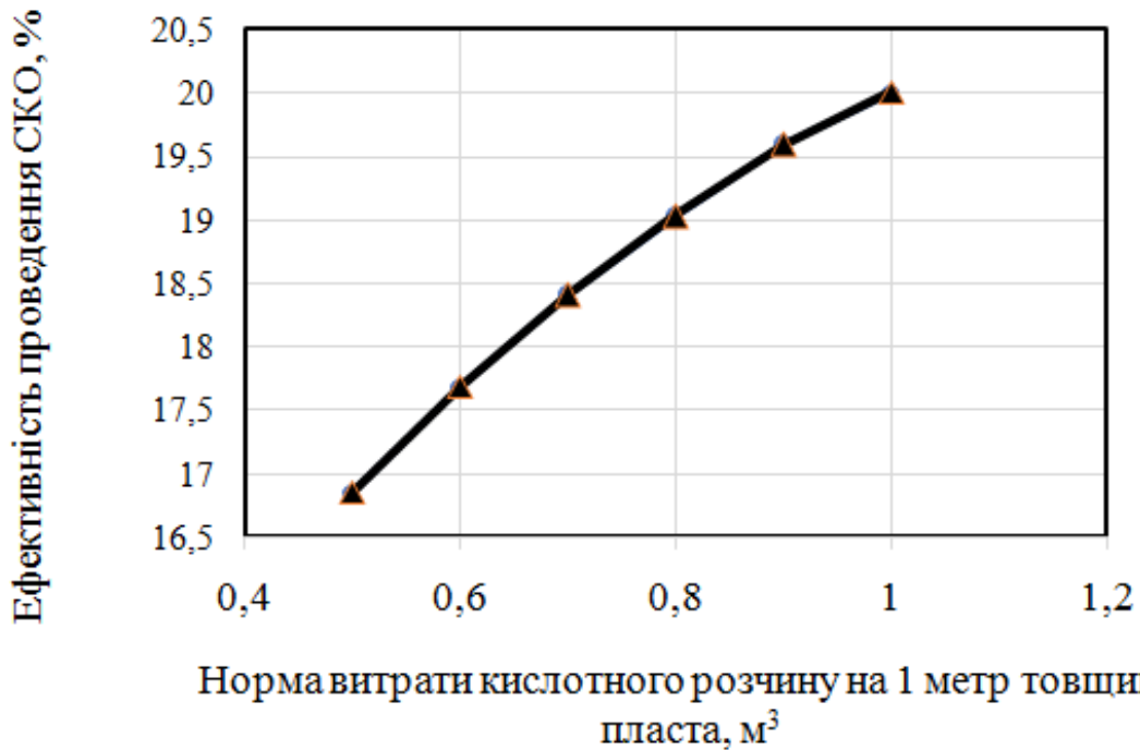
Рис 3. Залежність ефективності проведення солянокислотної обробки від норми витрати солянокислотного розчину на один метр товщини пласта
