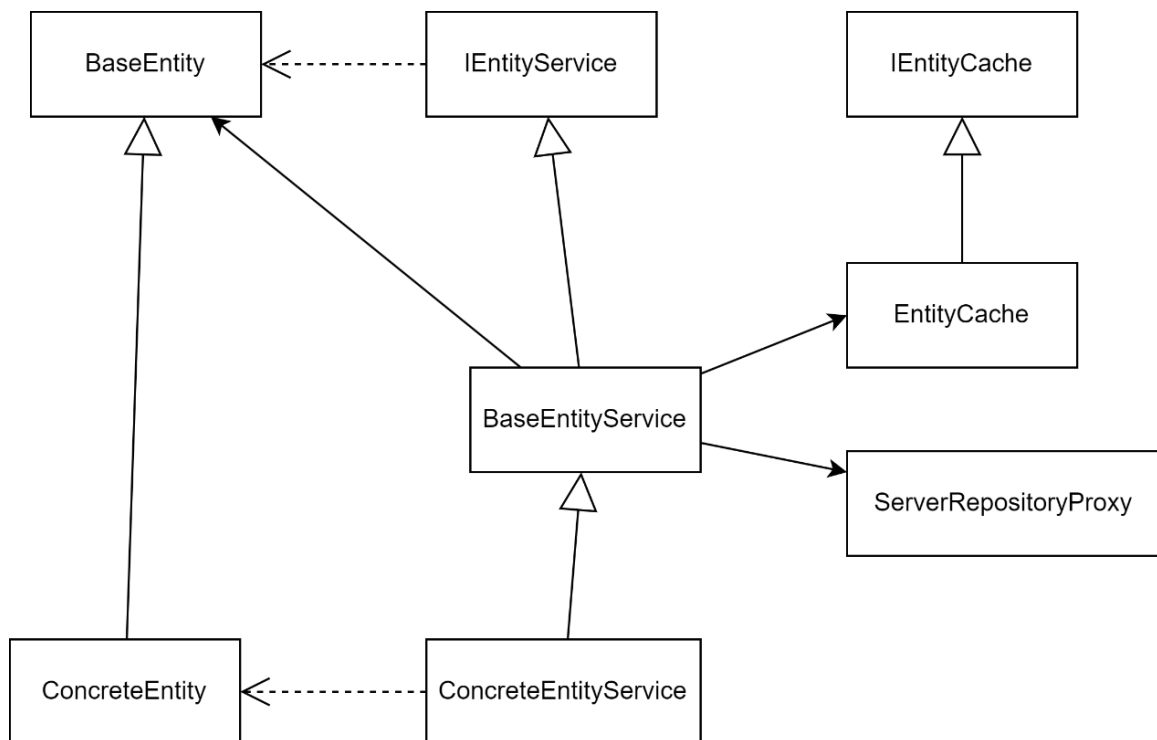
Рис. 1. Патерн ORM з підтримкою розподіленості
