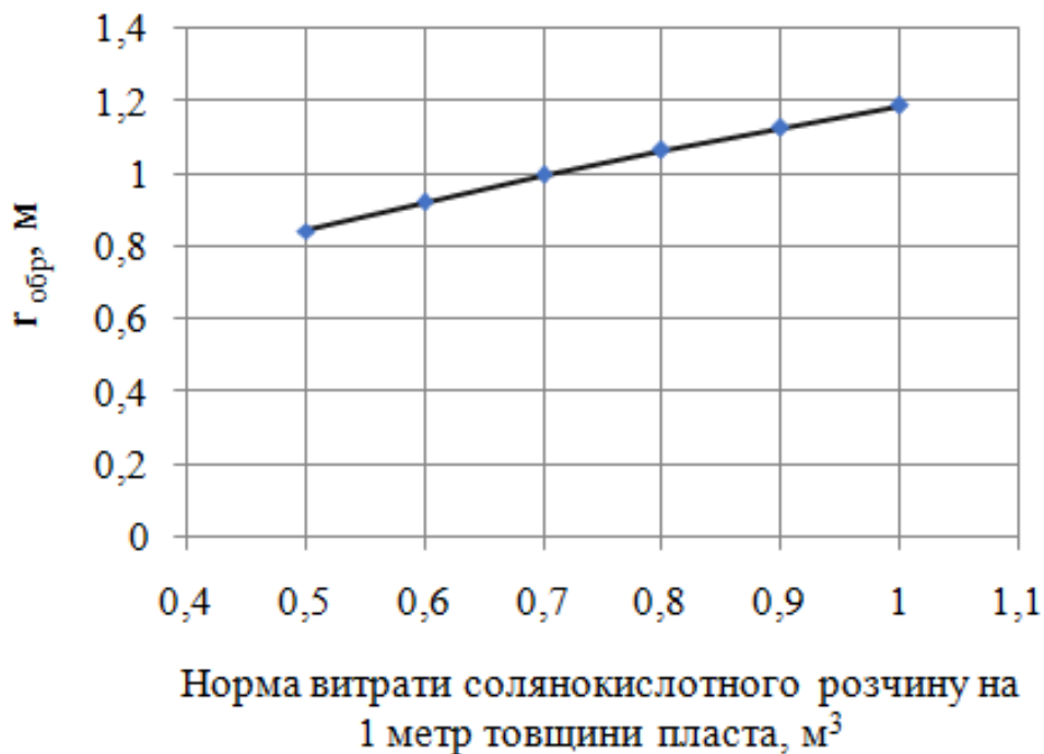
Рис 1. Залежність радіуса проникнення соляно-кислотного розчину від норми витрати розчину на один метр товщини пласта
