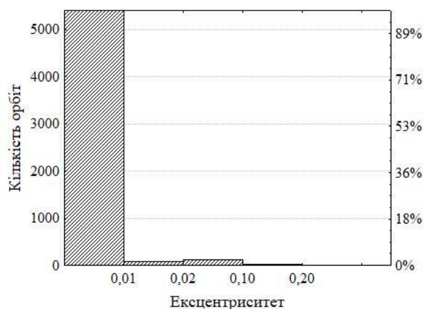
Рис. 1. Розподіл кількості орбіт НОО в залежності від ексцентриситету
