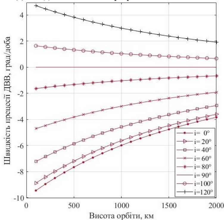
Рис. 4. Залежність швидкості прецесії ДВВ від висоти і нахилу орбіти
