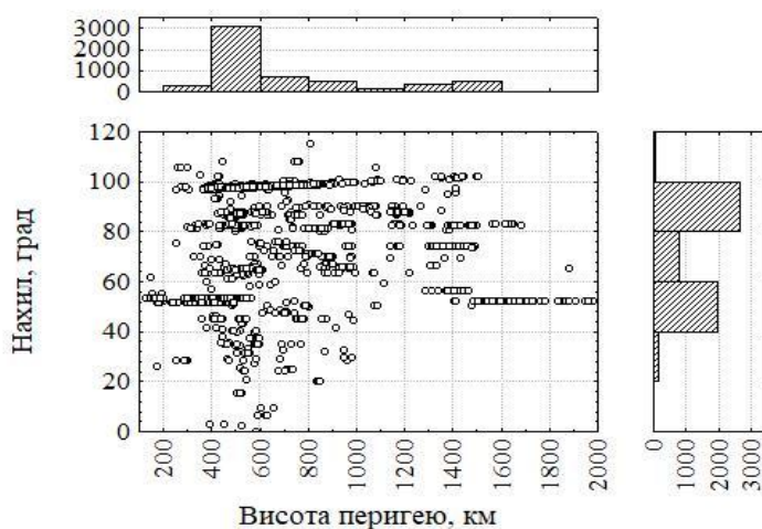
Рис. 2. Розподіл нахилу орбіт НОО в залежності від висоти перигею
