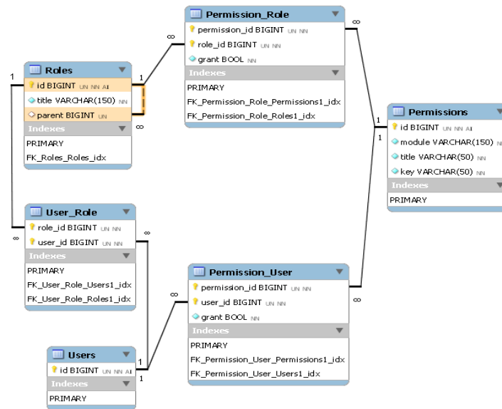
Рис.3. Схема реалізації ієрархічного відношення в MySQL
