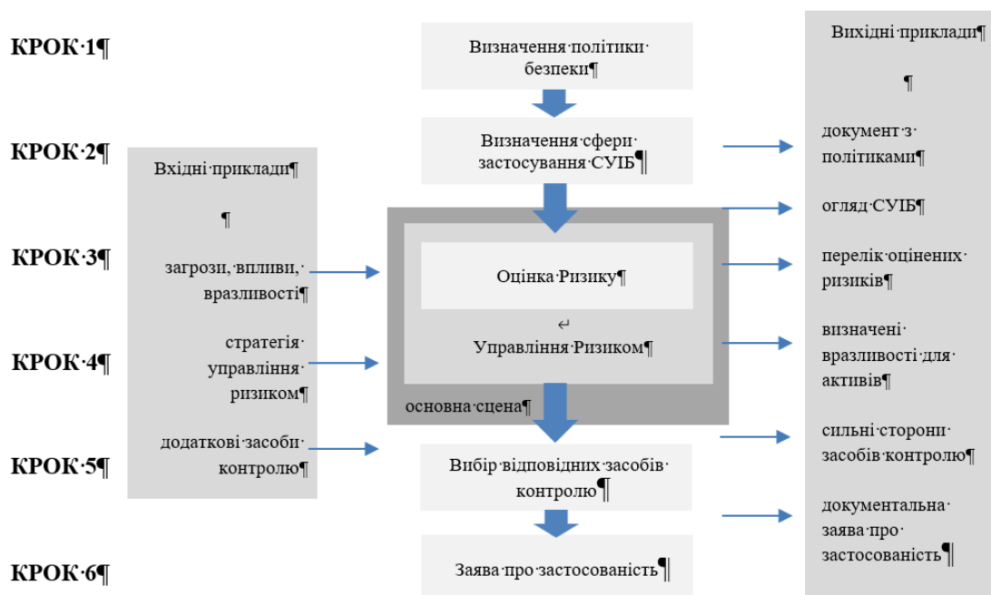
Рис. 3. СУІБ відповідно до фреймворку ISMS від ENISA [5, с.7]
